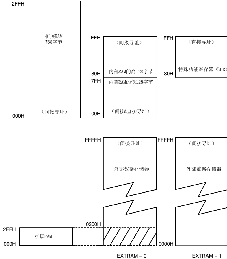
图6 内部和外部数据存储器结构
