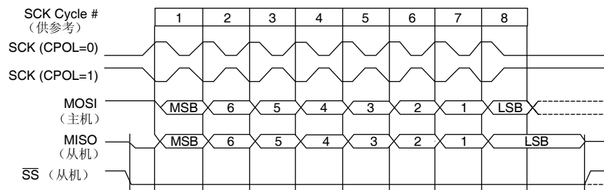
图 19 SPI 传输格式（CPHA=1）
