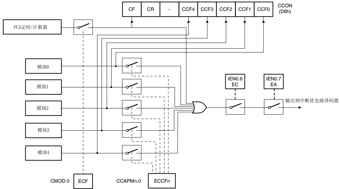
图 22 PCA 中断系统
