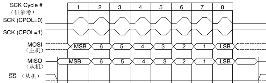
图 18 SPI 传输格式（CPHA=0）
