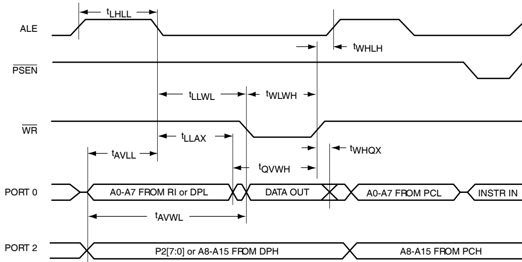
图 31 外部数据存储读周期
