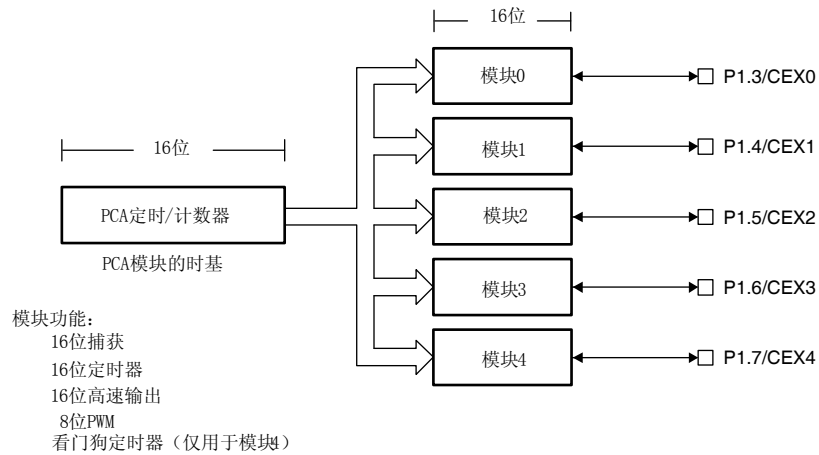
图 21 PCA 方框图
