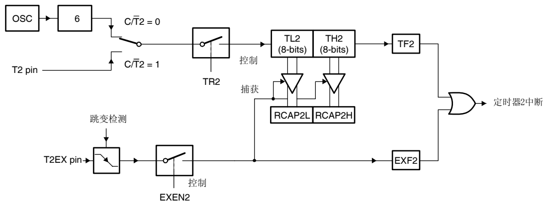
图 12 定时器 2 工作在捕获模式
