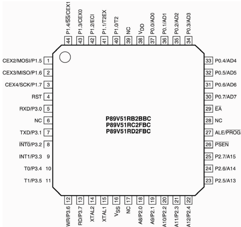
图 4 TQFP44 管脚配置
