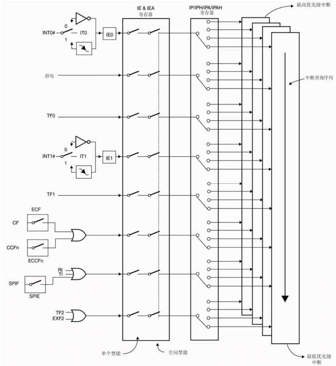
图 27 中断结构
